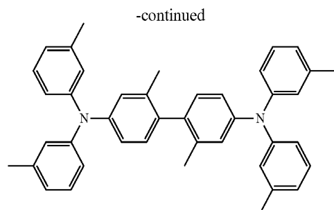
HMTPD
