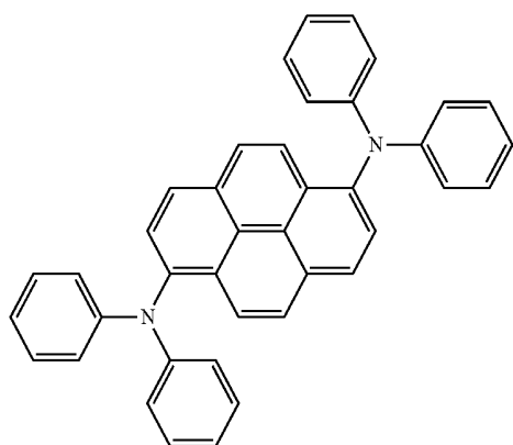
TPD
